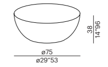
tavolo basso - low table TB-4
