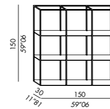
pensile - wall unit 150150 tre ripiani - three shelves
