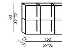
pensile - wall unit 150100 due ripiani - two shelves
