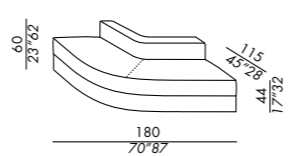
elemento elbow aperto - open elbow unit DEEP 180
