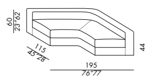
elemento elbow - elbow unit DEEP 195
