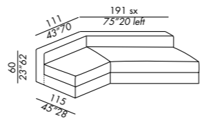
elemento asimmetrico - asymmetrical unit DEEP
