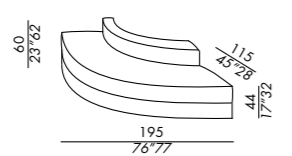
elemento curvo aperto - open round unit DEEP 195
