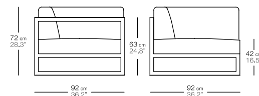
nude módulo esquinero corner module
