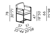
sedia - chair CINQUE WOOD
